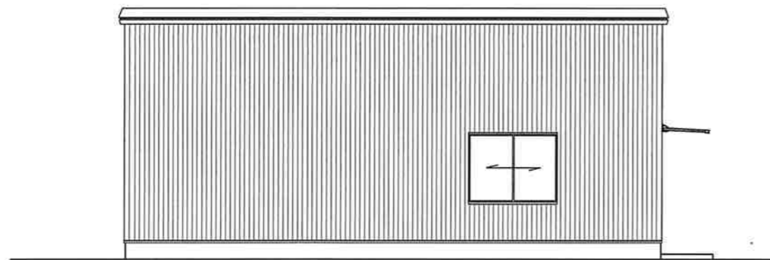
Y6 立面図 S=1/100
