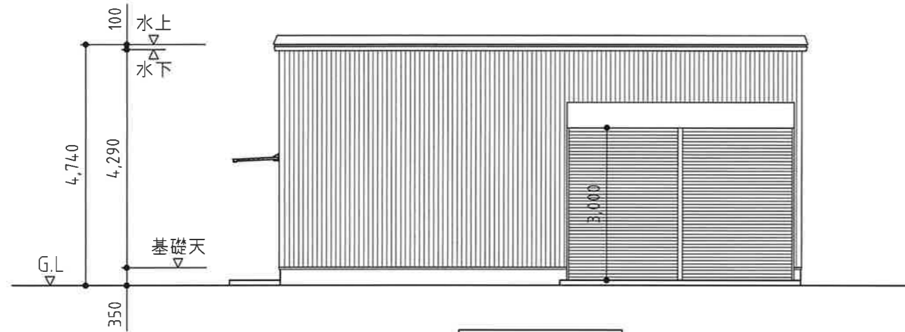
Y0 立面図 S=1/100
