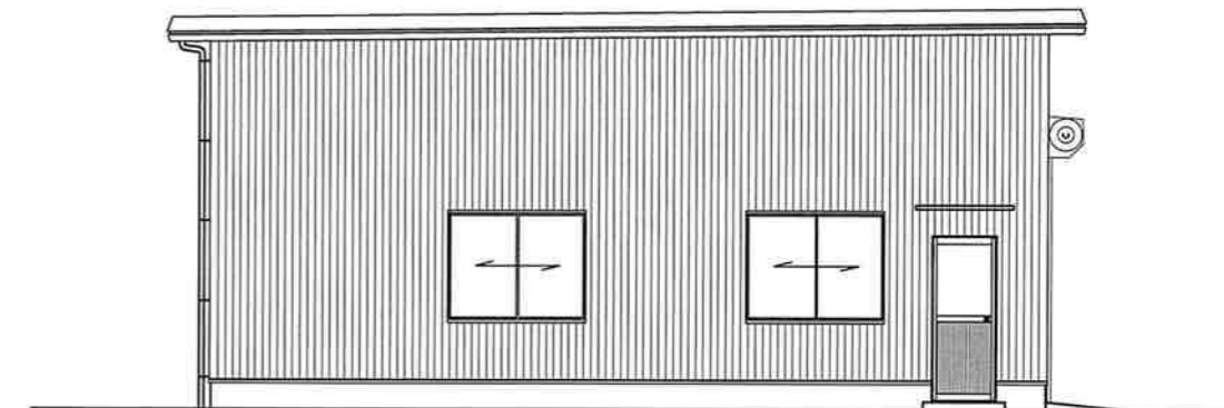
X0 立面図 S=1/100
