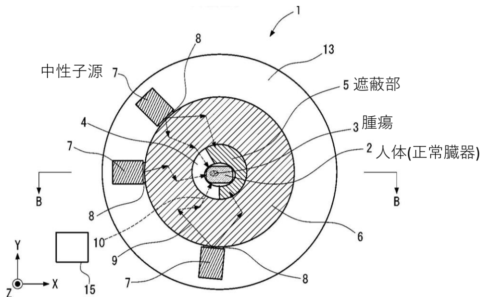
被曝抑制のため遮蔽部を有する 中性子捕捉療法装置の概念図
